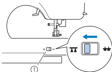
① Palanca de posición de dientes de arrastre
