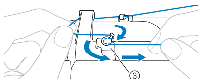
③ Guía de devanado de bobina
