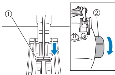
① Orificio en la placa de la aguja ② Rueda
